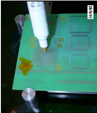
Nanoszenie topnika
