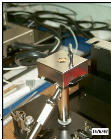
1. Operacje zakładania maski z otworami, 2. Usuwania nadmiaru kulek, 3. Zamykania piecyka
