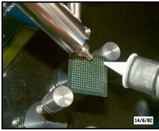
Usuwanie resztek spoiwa z US.
